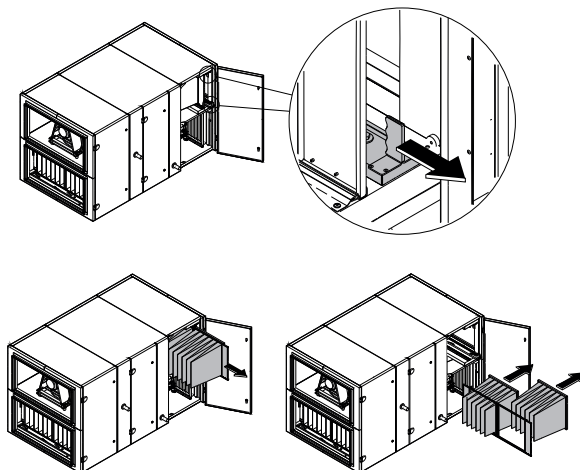
Abb. 3. Filter-Klemmvorrichtung
